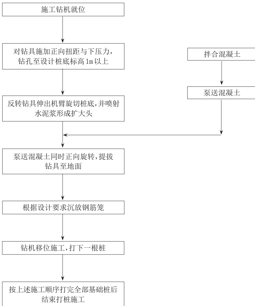
图B.0.3 出土30%挤土机械扩底灌注桩施工工艺流程框图
