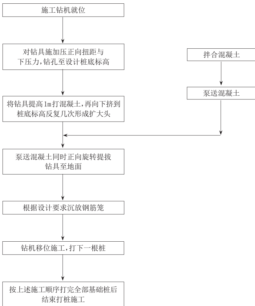
图 B.0.4 螺旋钻具挤压扩底成型桩施工工艺流程框图
