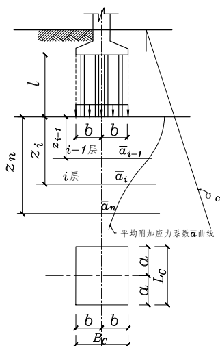
图 5.3.10 桩基沉降计算示意图
