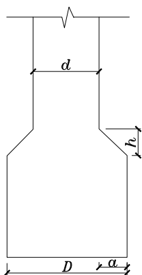
图4.5.5 扩底桩构造
