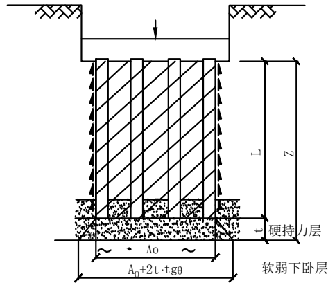
图 5.3.1 软弱下卧层承载力验算
