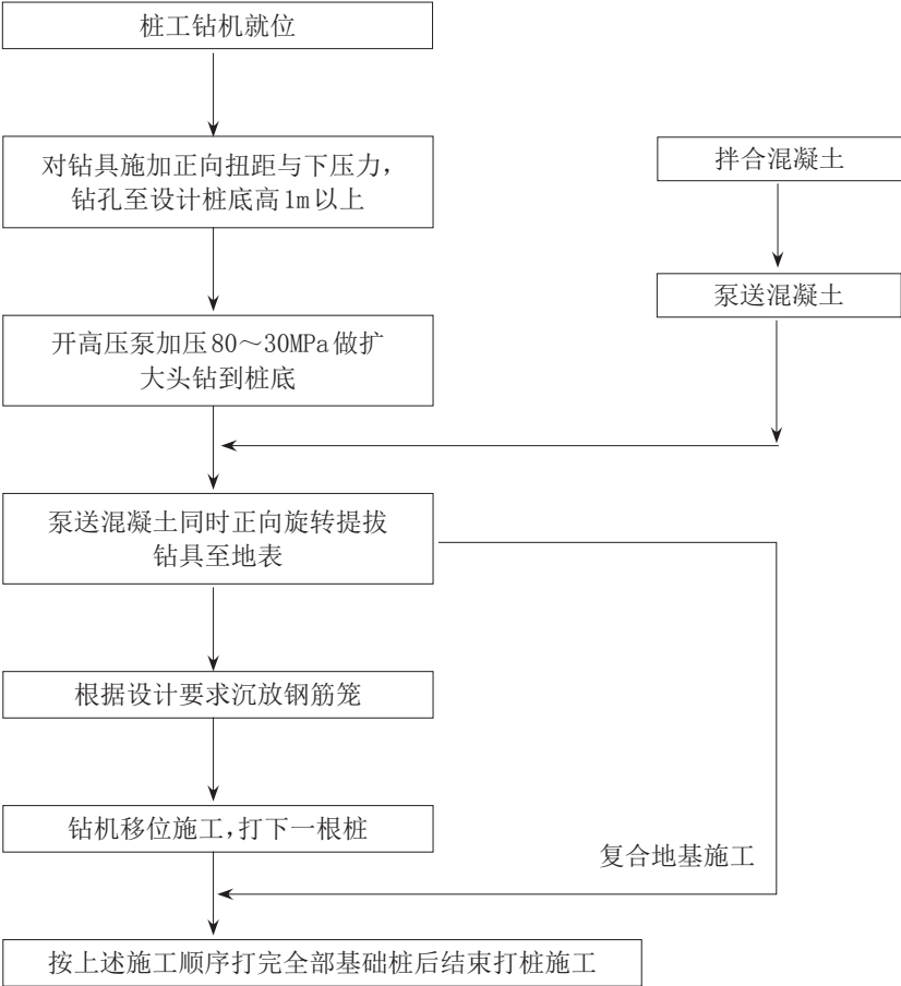
图 B.0.1 螺旋挤土扩底灌注桩施工工艺流程框图
