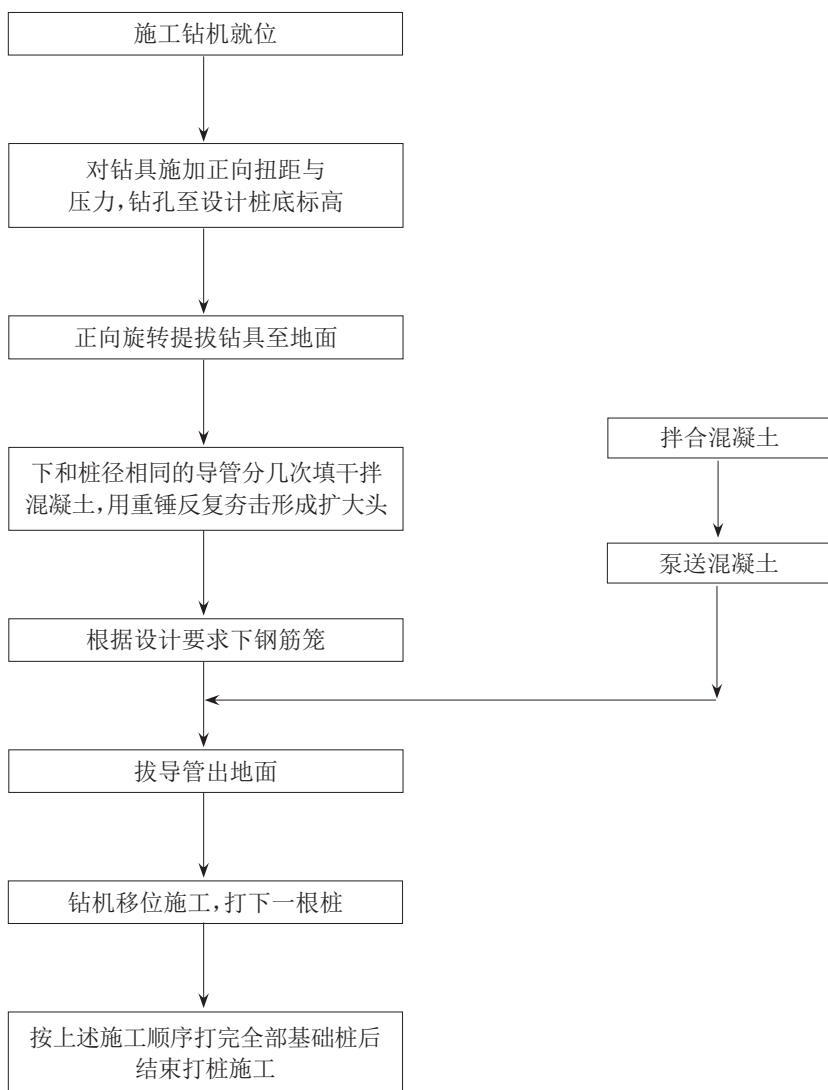
图 B.0.2 螺旋挤土夯击扩底灌注桩施工工艺流程框图
