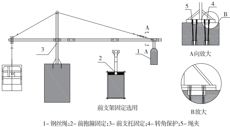
图4.3.7 FCG05安装图示
