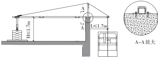
图 4.3.3 FCG01 安装图示
