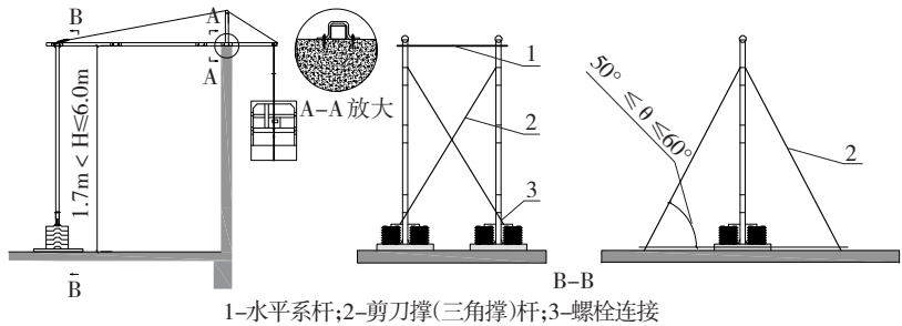
图 4.3.5 FCG03 安装图示
