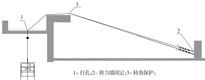
图 4.3.8 FCG06 安装图示
