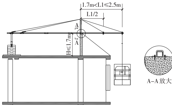
图 4.3.4 FCG02 安装图示
