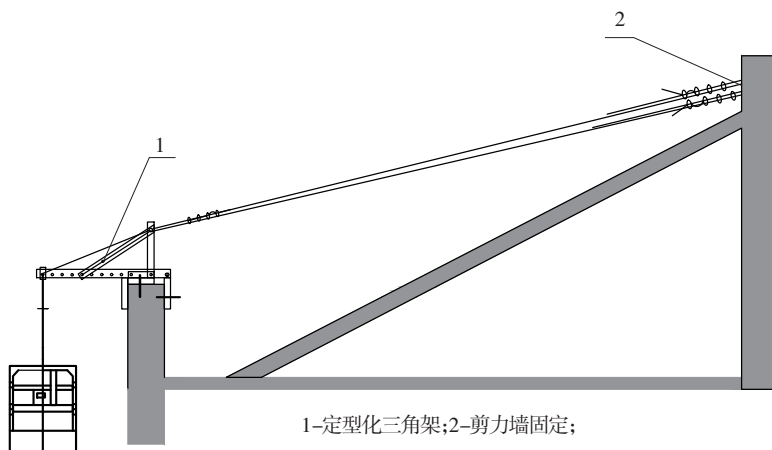
图 4.3.9 FCG07 安装图示
