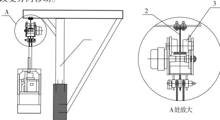
图 4.3.10 FCG08 安装图示
