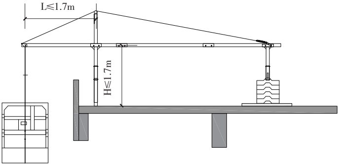
图 4.2.1 悬挂装置常规安装图示
