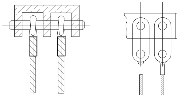
图 5.0.11 典型悬挂点示例
